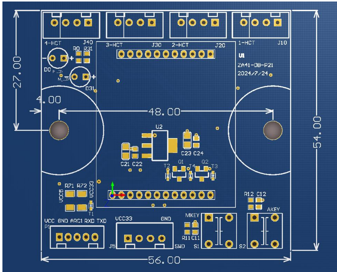
图 1：底板尺寸图(定位孔径为 4.2mm)
